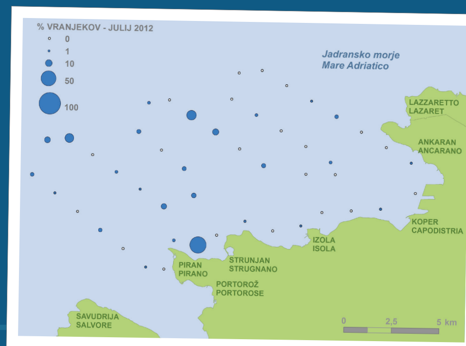
Zemljevid 2: Popisi sredozemskih vranjekov in drugih morskih ptic na morju razkrivajo, kje so najpomembnejša območja za njihovo prehranjevanje.
