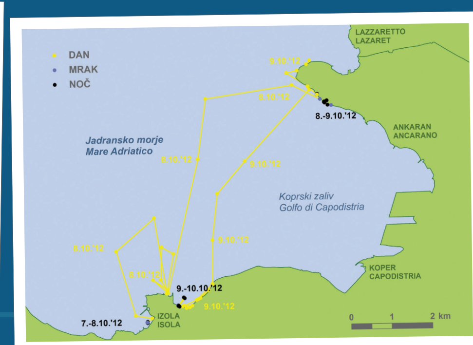
Zemljevid 3: Spremljanje posameznih osebkov z GPS sledilnimi napravami omogoča določanje njihovih dnevnih poti na slovenskem morju.
