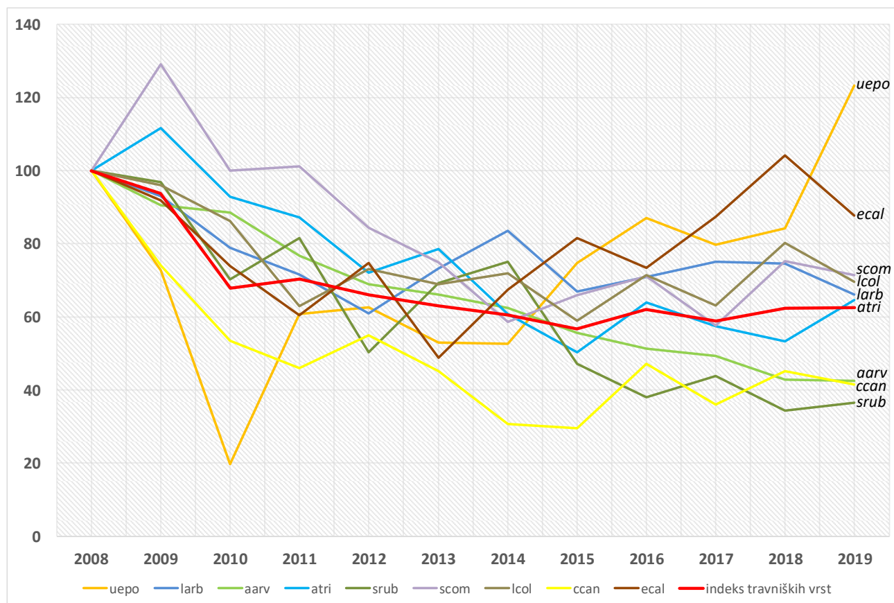
Slika 4: Indeksi travniških vrst ptic v letih 2008-2019; uepo – smrdokavra, larb – hribski škranec, aarv – poljski škranec, atr – drevesna cipa, srub – repaljščica, scom – rjava penica, lcol – rjavi srakoper, ccan – repnik, ecal – veliki strnad; rdeča črta – sestavljeni indeks
